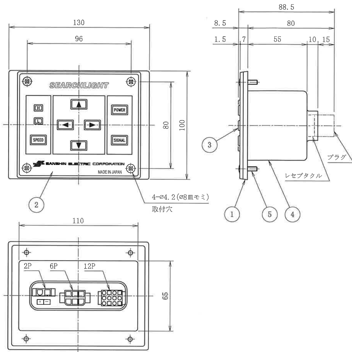
裏面図
